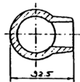
End post nr. 2005-4 C, section Z-Z
