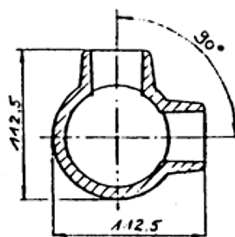
Schnitt Y-Y
