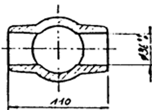
Middle post nr. 2005-4 A, section Z-Z
