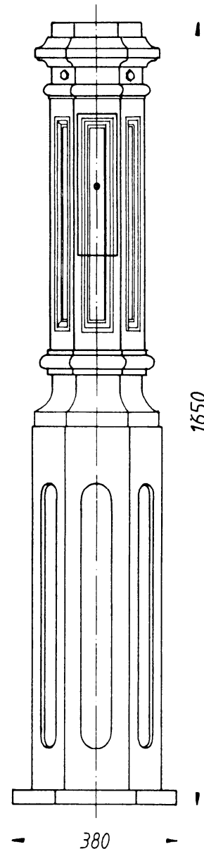
THK-610-E Kandelaber-Unterteil mit Tür zum Eingraben Gewicht: ca. 124,5 kg
