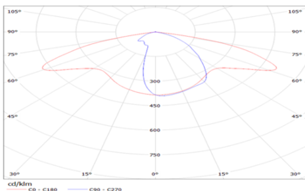
Diagramme polaire
